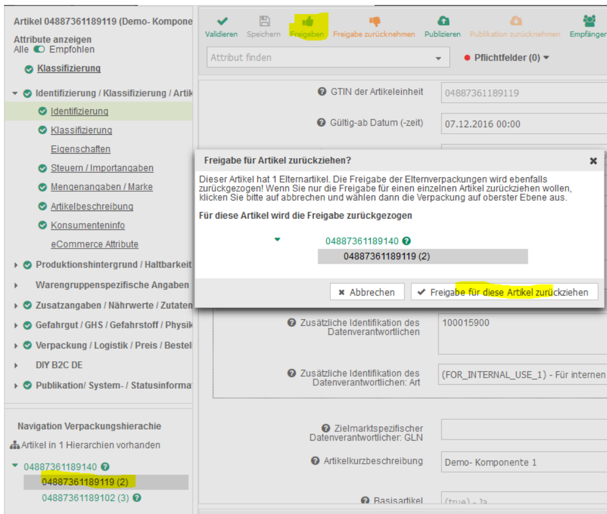
Abbildung 85: Anwendungsbeispiel, Bearbeiten einer publizierten Hierarchie – Freigabe zurücknehmen
