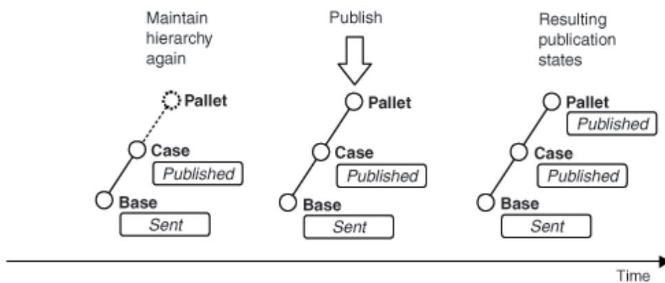
Abbildung 161: Spätere Publikation einer nachträglichen Erweiterung einer einfachen Hierarchie
