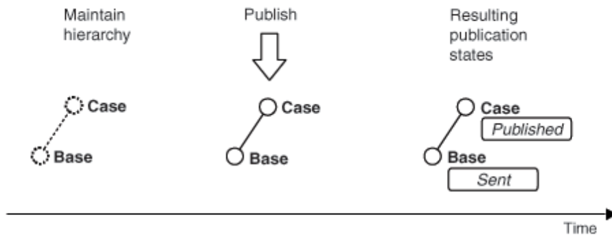
Abbildung 160: Bearbeitung und Publikation einer einfachen Hierarchie
