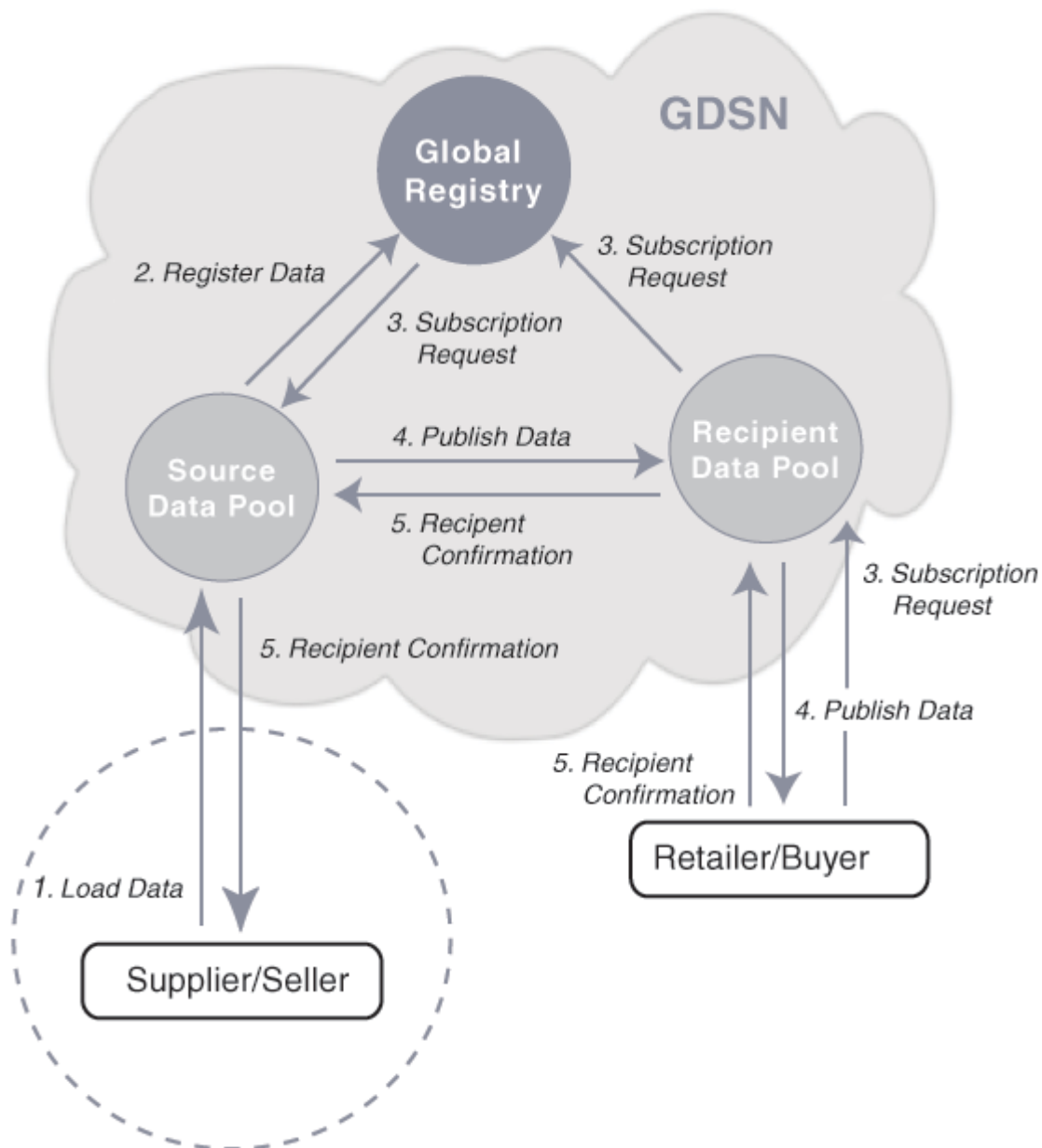
Abbildung 2: GDSN-Choreografie
