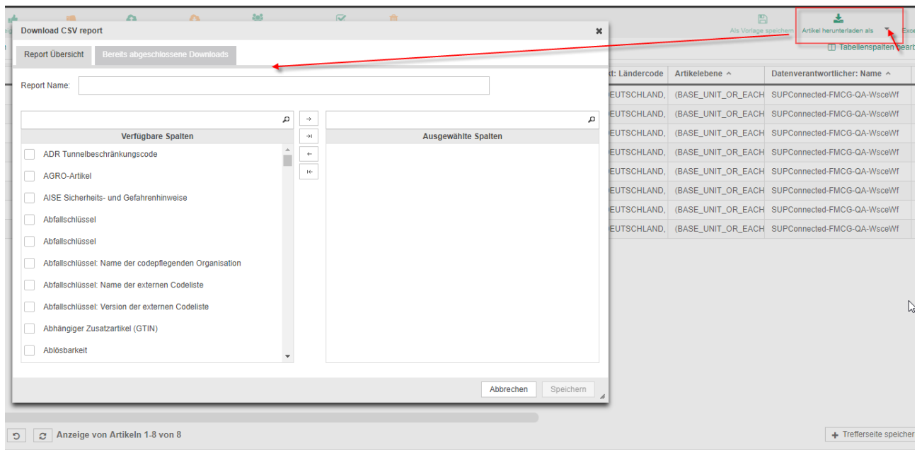
Abbildung 36: CSV-Report konfigurieren
