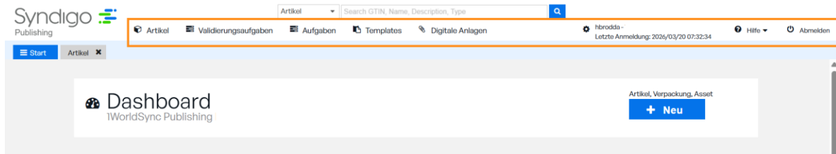
Abbildung 18: Menüstruktur
