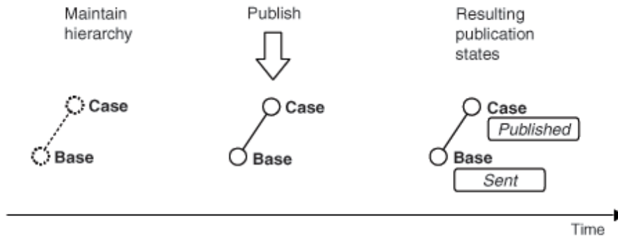
Abbildung 172: Bearbeitung und Publikation einer einfachen Hierarchie
