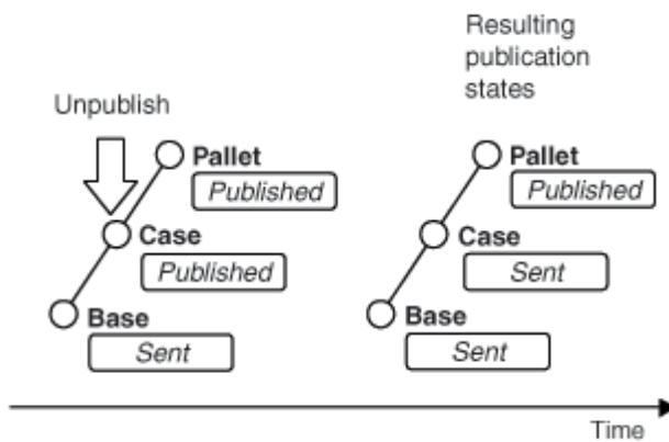
Abbildung 174: Zurücknahme der Publikation für einen Teil der Hierarchie
