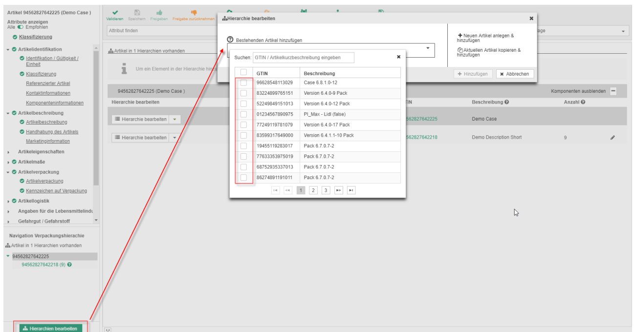
Abbildung 88: Hierarchien bearbeiten, Bestehenden Artikel hinzufügen
