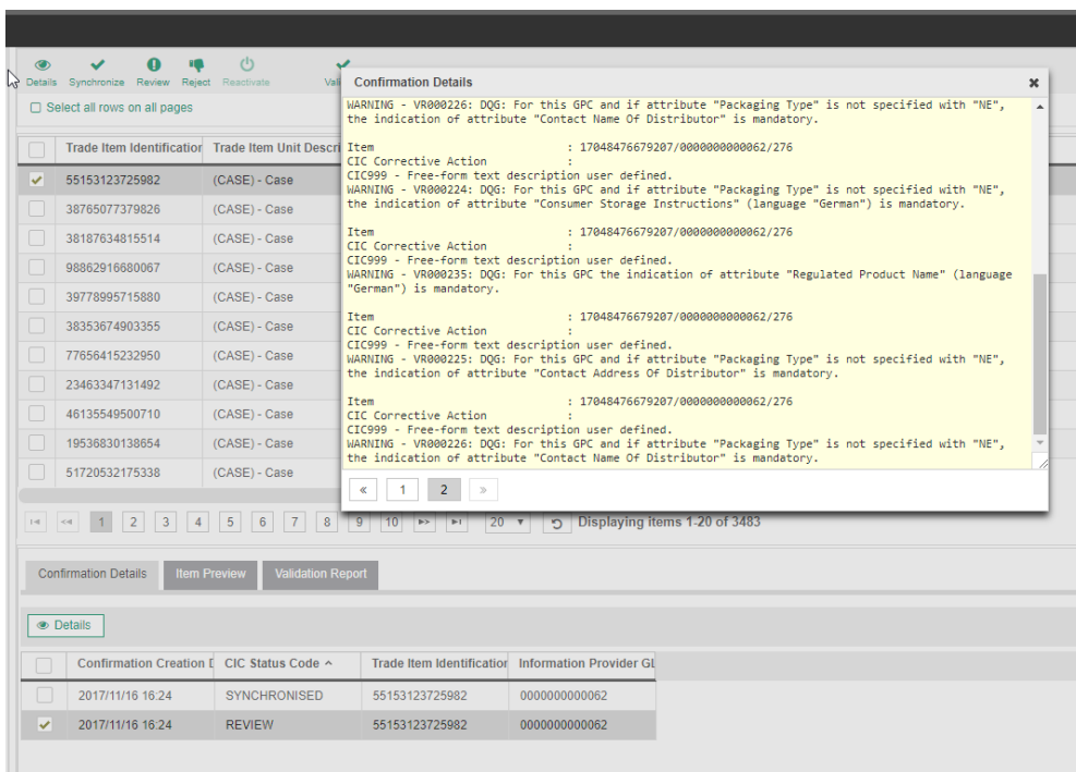
Abbildung 55: Confirmation Details, Korrekturmaßnahmen
